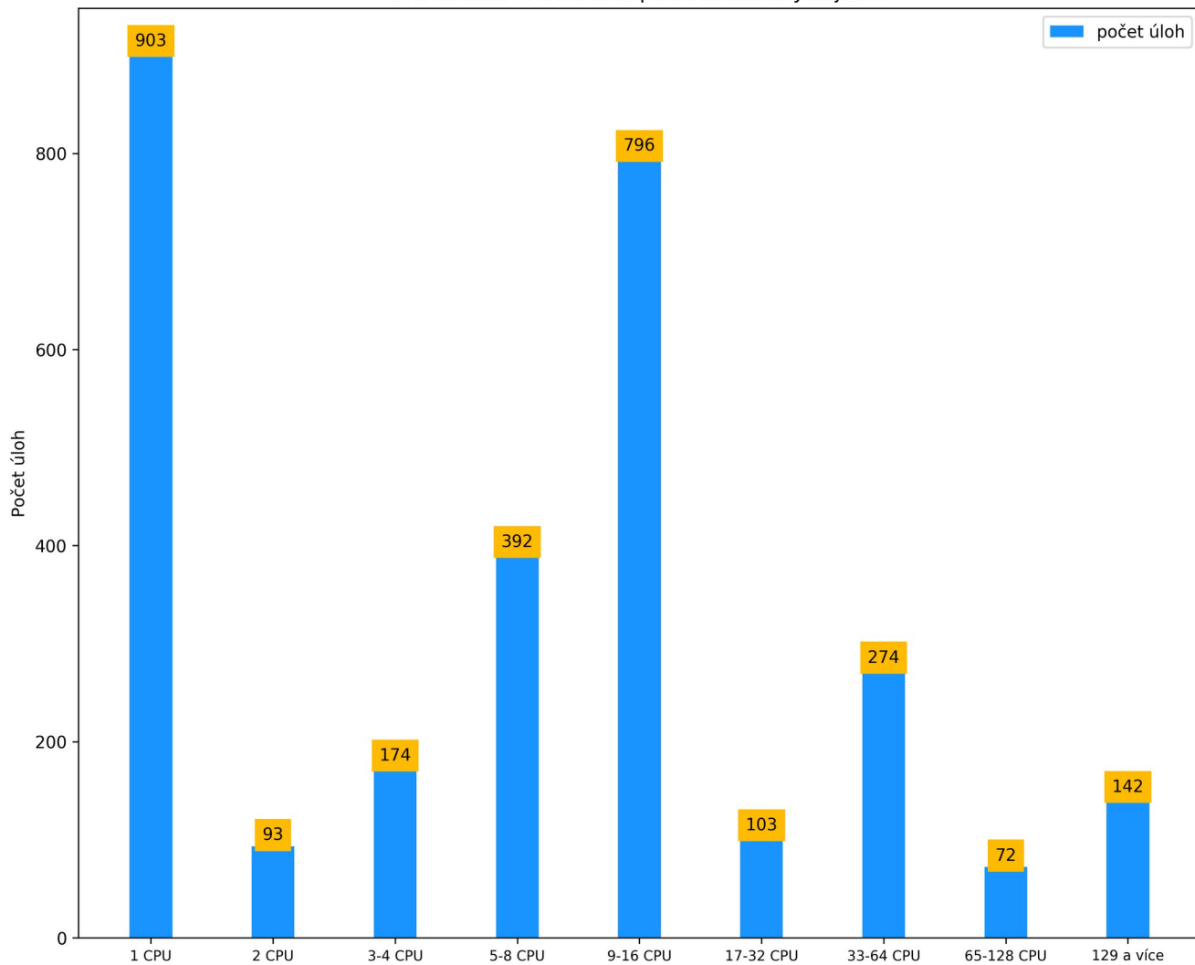
Fronta luna - Počet úloh podle alokovaných jader
